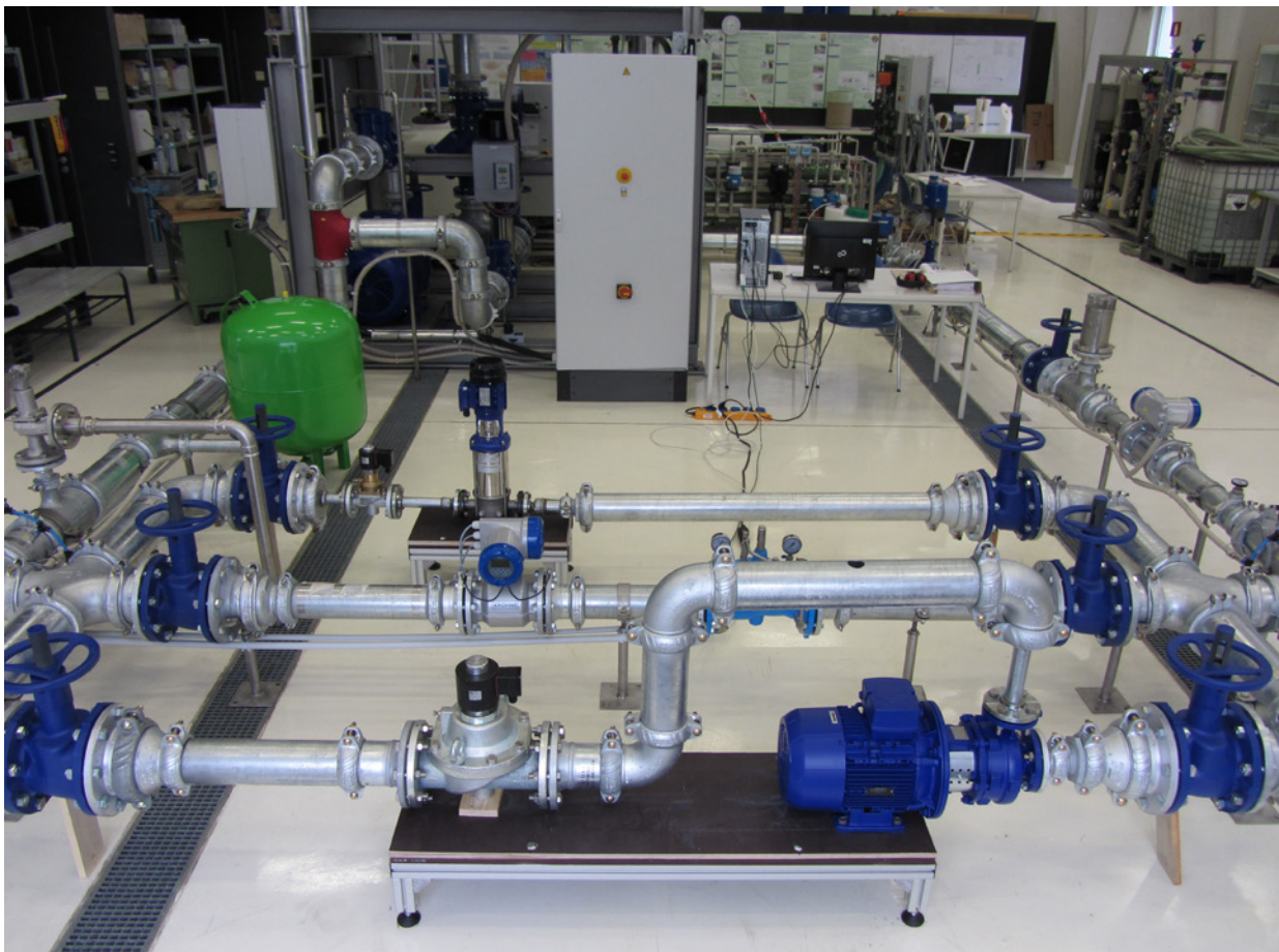
Bild 1: Prüfstand an der UniBwM zur Simulation verschiedener Wasserversorgungsszenarien inkl. unterschiedlicher PaTs.
