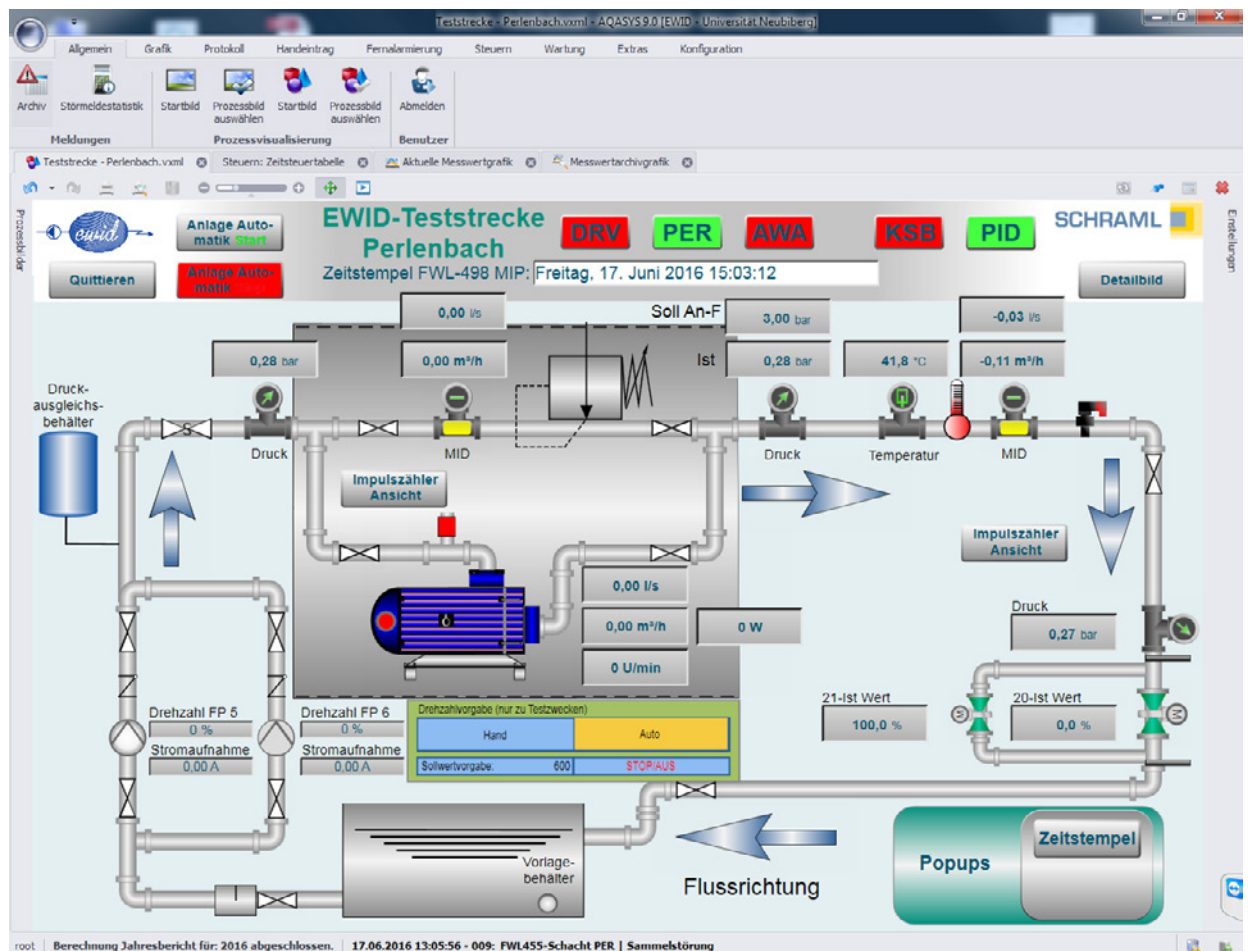
Bild 2: Im Prozessleitsystem laufen alle Parameter zusammen. Die intelligente Druckregelung ist von hier aus leicht zu überwachen und bedienen.
