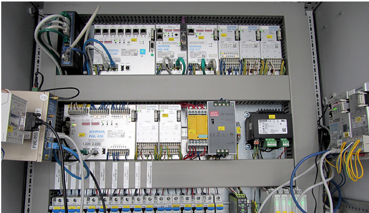
Bild 3: Sogenannte SPS-Fernwirkstationen übertragen ihre Daten nahezu in Echtzeit an das Prozessleitsystem.
